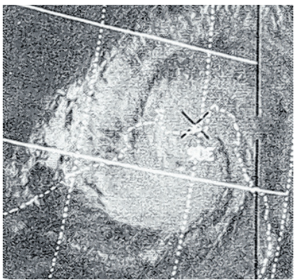
Satelitska slika ciklona Bhola
