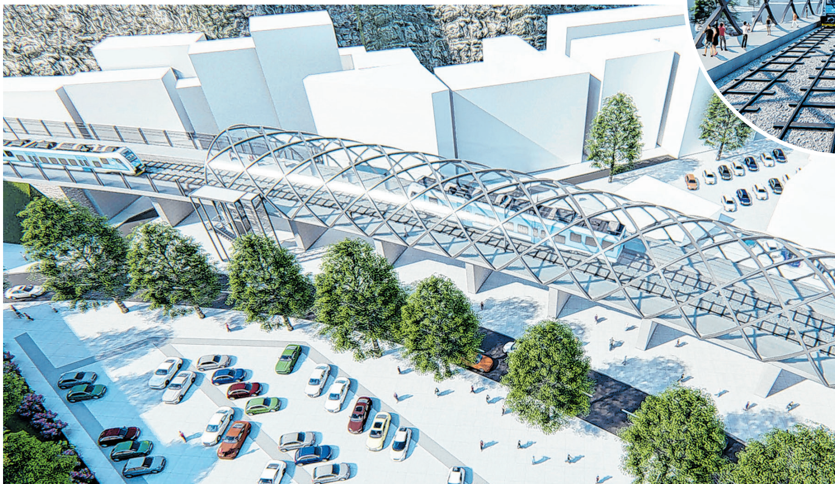
Novi željeznički most na Školjiću, na mjestu sadašnjeg nasipa i manjeg mosta, bit će dugačak 255 metara
